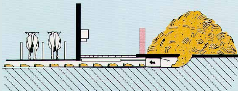
Presse -tlakové odstraňovanie hnoja
